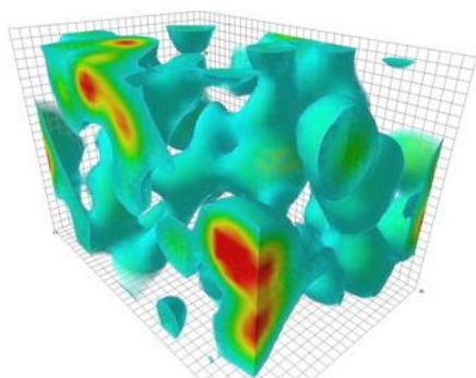
Флуктуации вакуума.
